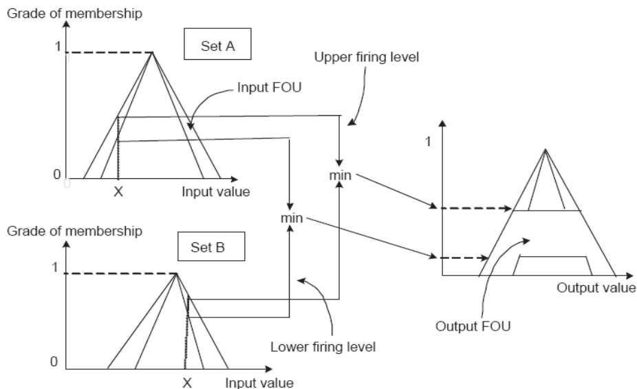
Fig. 4. IT2 FL calculation of output FOU
