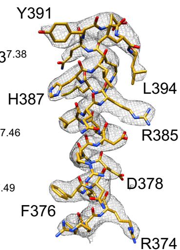
GαRas α5
