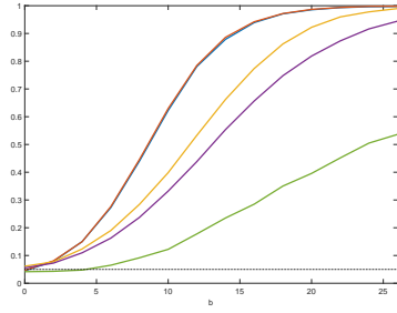
(d) \tau = 0.2 , DGP2a - GARCH(1,1)
